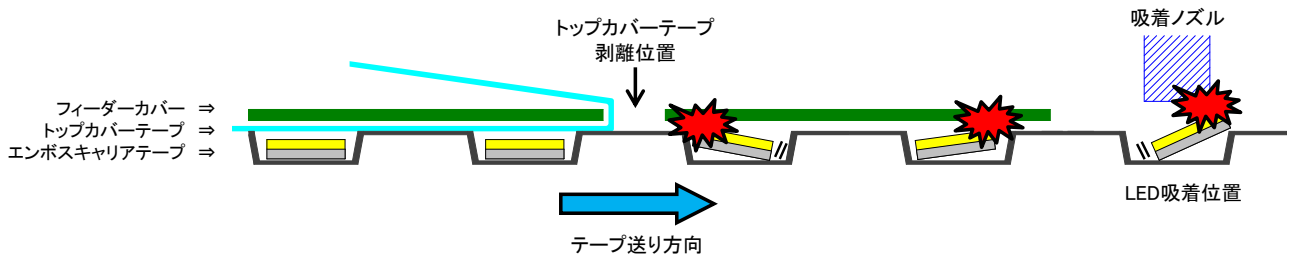
図 20. テープ送りによる不具合例
