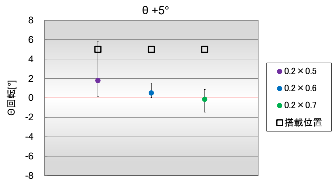
図 11. NCSxE17A 試験結果( \theta +5°)
