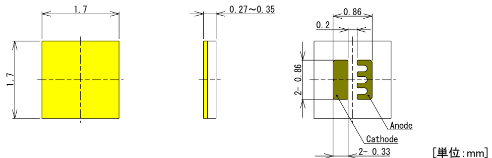
図 3. NCSxE17A 外形寸法
