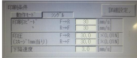
図 18. 印刷条件設定例
