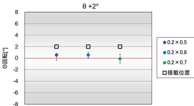
図 10. NCSxE17A 試験結果( \theta +2°)
