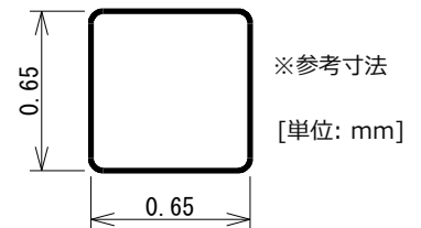
図 21. 吸着ノズル参考例
