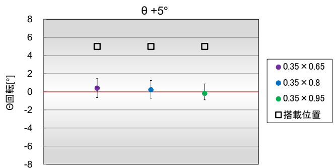
図 15. NVSxE21A 試験結果 ( \theta + 5^\circ )
