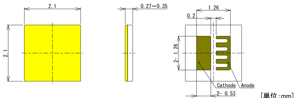
図 4. NVSxE21A 外形寸法
