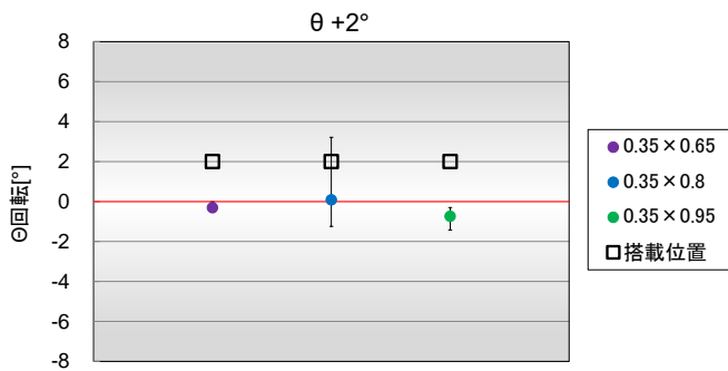
図 14. NVSxE21A 試験結果 ( \theta + 2^\circ )
