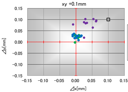
図 8. NCSxE17A 試験結果(xy+0.1mm)
