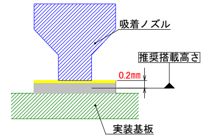
図 24. 推奨搭載高さ
