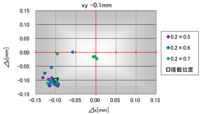
図 9. NCSxE17A 試験結果(xy-0.1mm)
