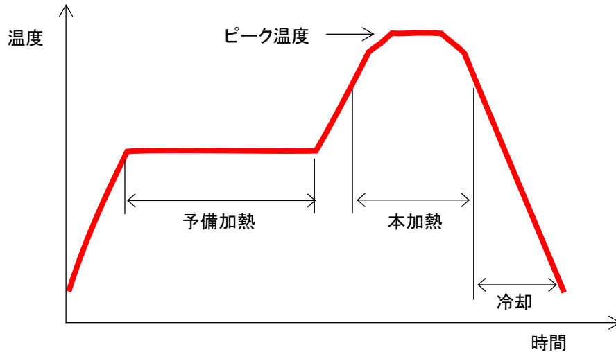
図 25. リフロープロフィール
