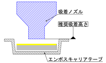
図 23. 推奨吸着高さ
