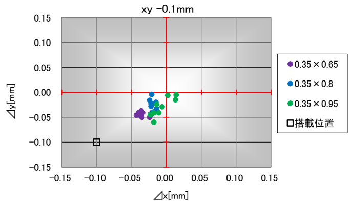
図 13. NVSxE21A 試験結果 (xy-0.1mm)
