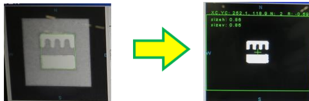
図 22. 吸着時の部品認識、補正例
