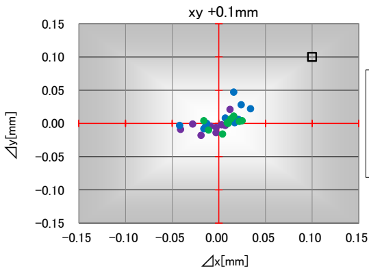
図 12. NVSxE21A 試験結果 (xy+0.1mm)
